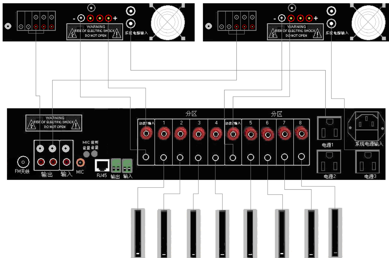
(11) 接线图:
