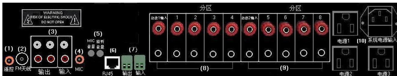
(11) 接线图:
